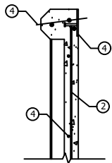
3 TOP AND BOTTOM EDGE DETAIL
